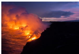
希洛岛-基拉韦厄火山
